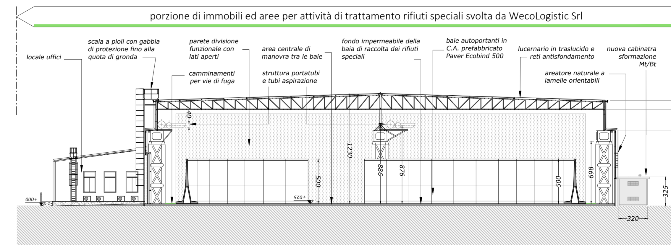
SEZIONE TRASVERSALE CC' - VISTA GENERALE SCALA 1:250
